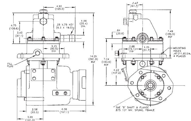
GB60 • CLUTCH SHIFT
