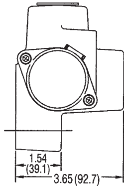
LEVERSHIFT KNOB
